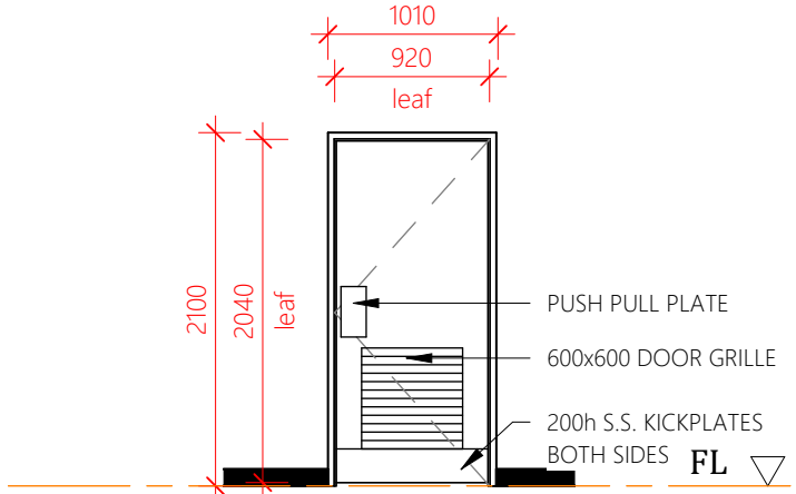
DOOR TYPE G
