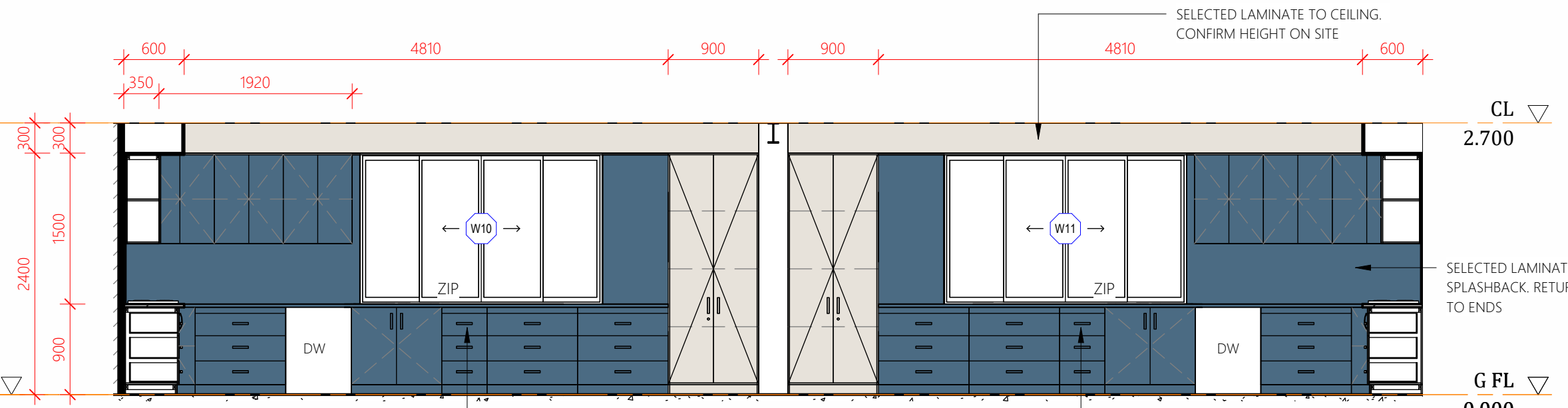
Elevation 2B
