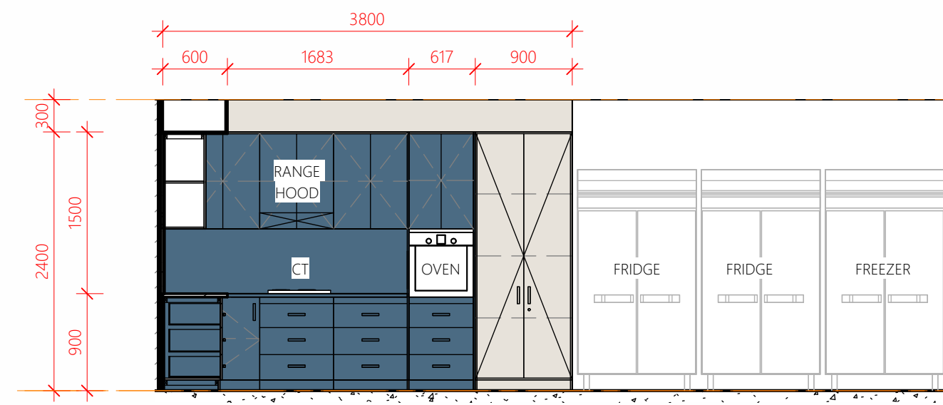
Elevation 2A
