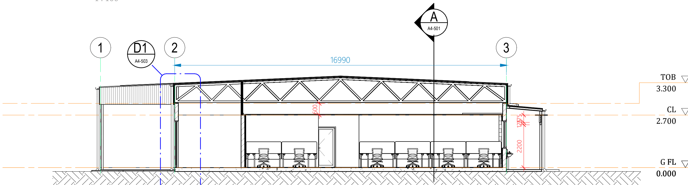
SECTION D 1 : 100
