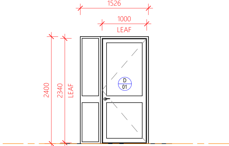
DOOR TYPE A
