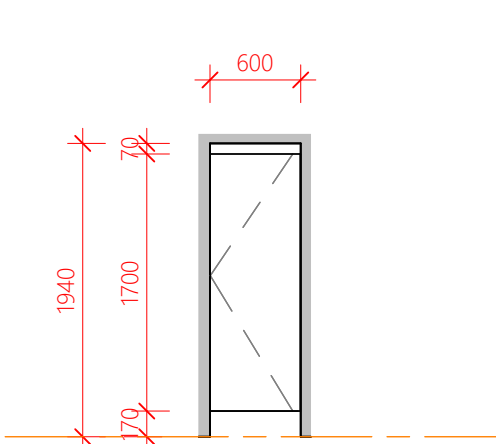
DOOR TYPE K
