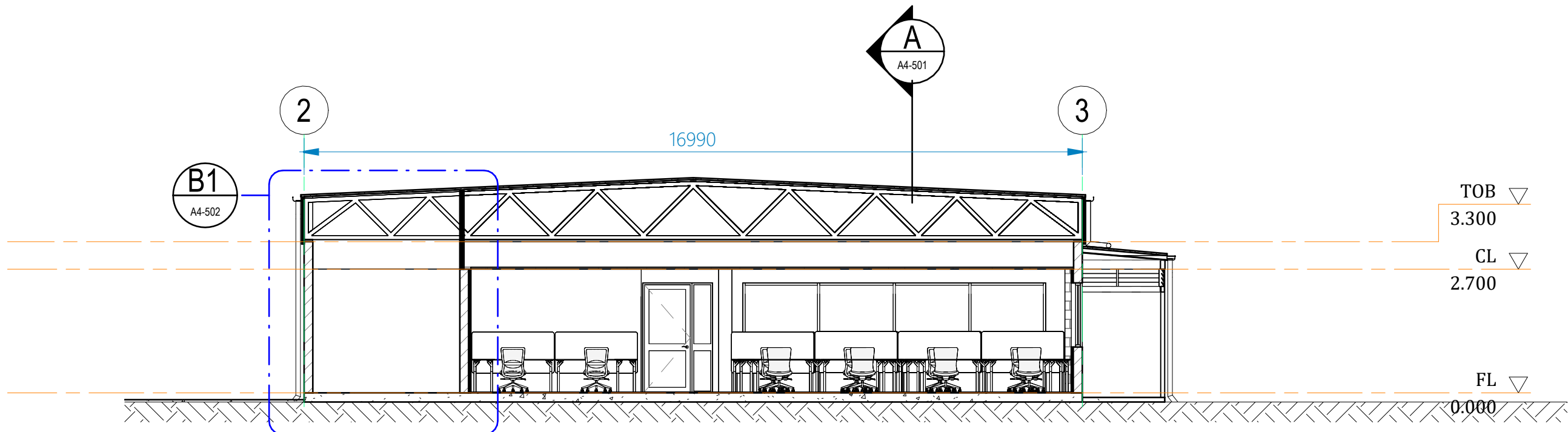
SECTION B 1 : 100
