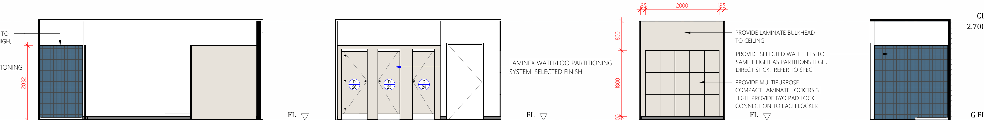
Elevation 4J
