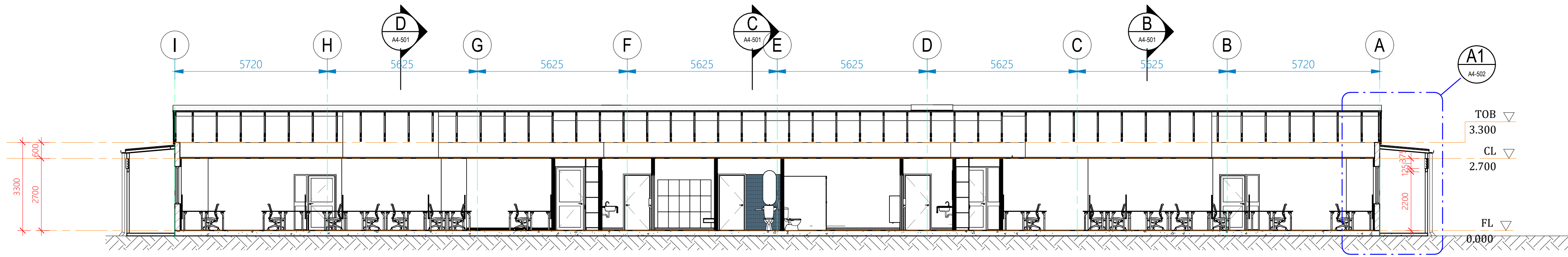
SECTION A 1 : 100
