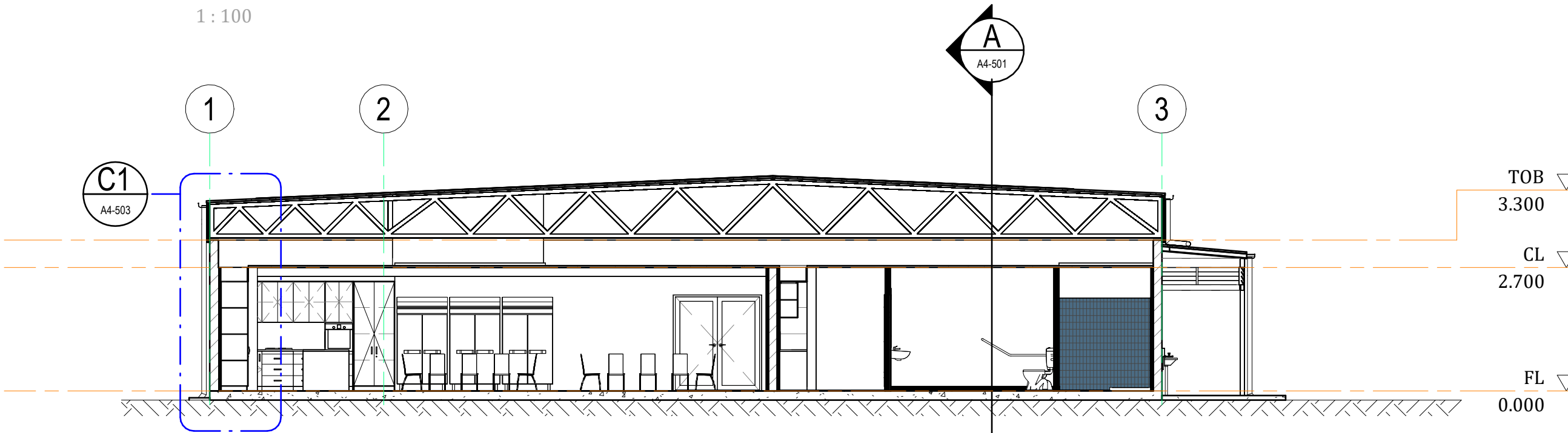
SECTION C 1 : 100
