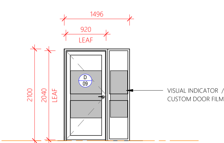
DOOR TYPE D
