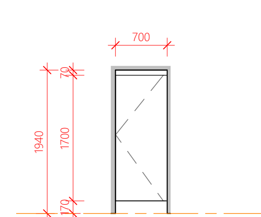
DOOR TYPE J
