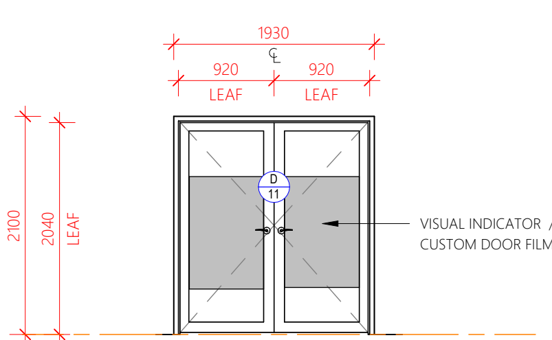
DOOR TYPE C
