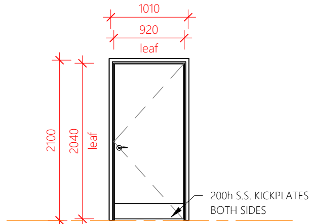
DOOR TYPE H
