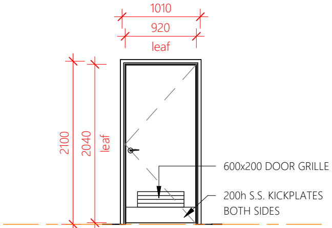
DOOR TYPE F
